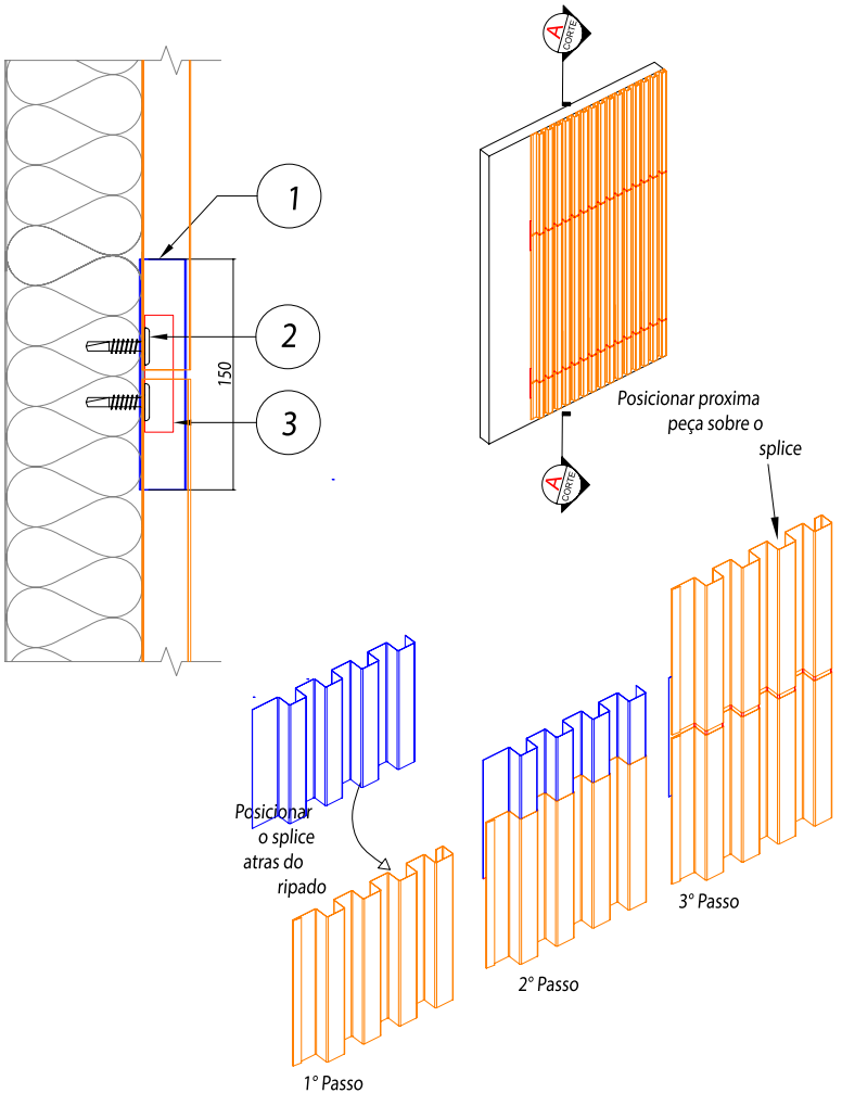
Detalhe de emenda com splice
