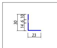
Acab inferior de montagem com início suspenso
