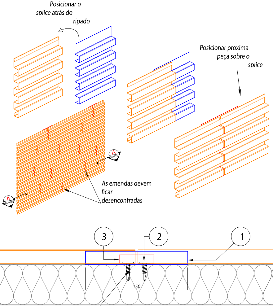
Detalhe de emenda com splice detalhe em painel
