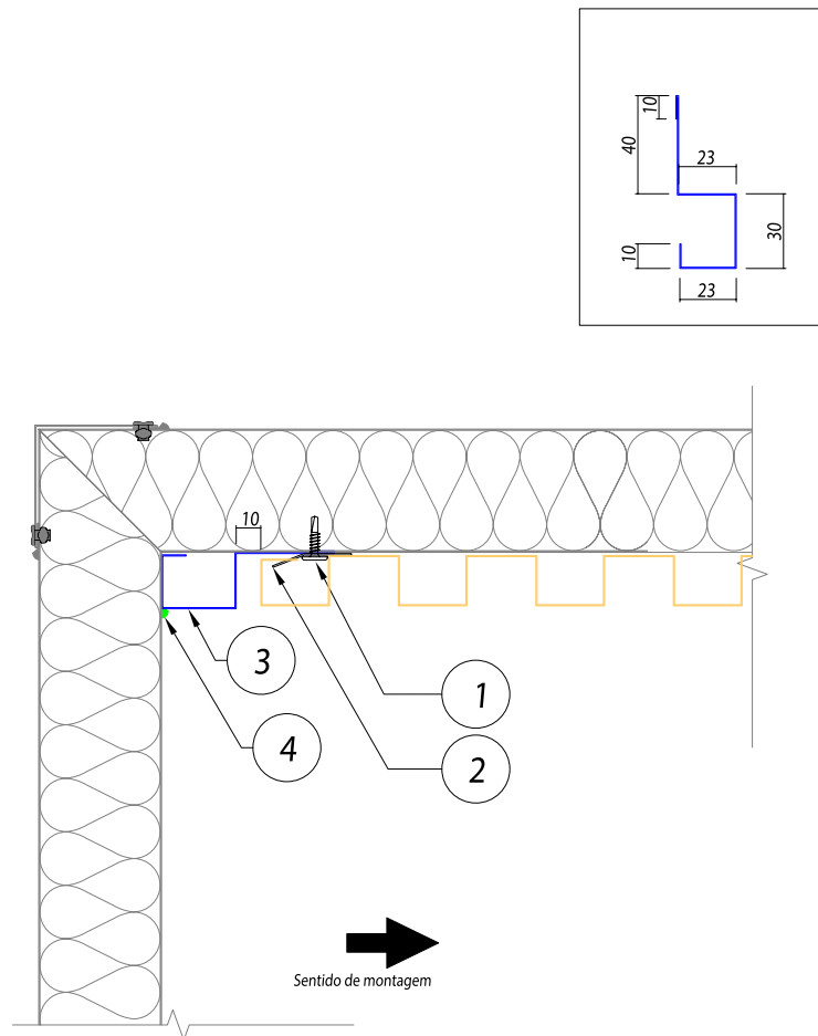
Acabamento com encontro com painel
