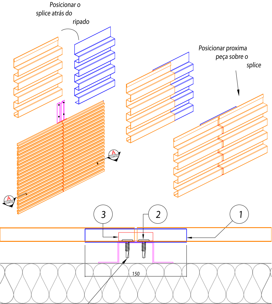
Detalhe de emenda com splice Detalhe em perfil metálico
