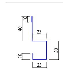
Acabamento inferior de montagem
