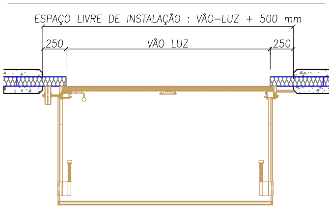
VISTA SUPERIOR
