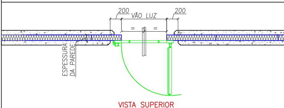
VISTA SUPERIOR
