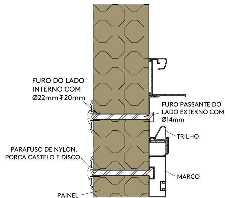
SEÇÃO A-A
