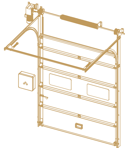
PERSPECTIVA
